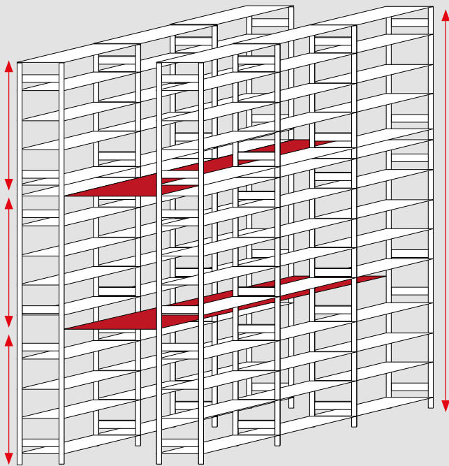
Legbordenmagazijn met 3 etages
