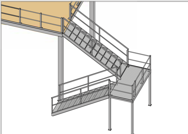
Dubbele trappen in tegengestelde richting met draaiplatform
