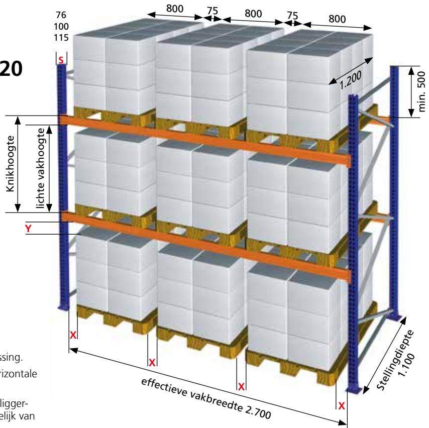
Voorbeeld: europallet zonder overhang
