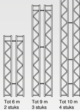
Aantal koppelstukken in de hoogte
