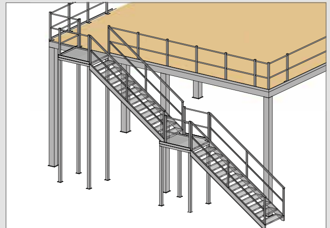
Dubbele rechte trappen met tussenplatform
